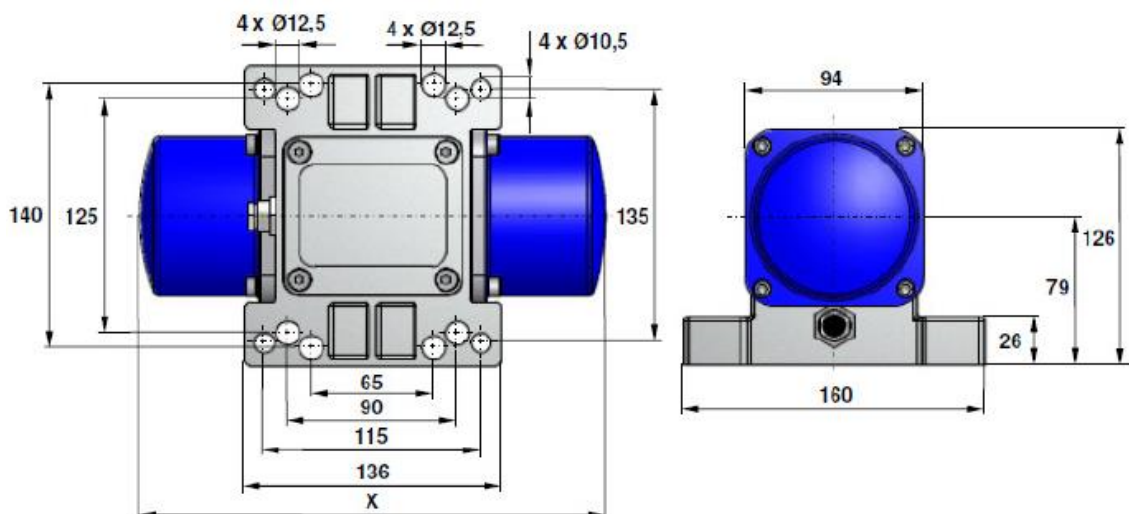
Abbildung 2 Abmaße
