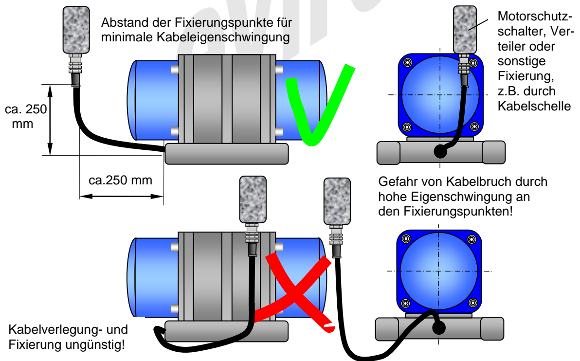
Abbildung 5 Kabelverlegung Anschlussleitung
