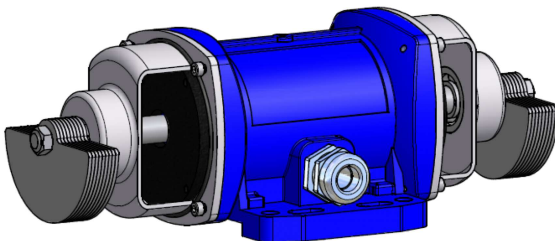
Abbildung 6 Einstellung der Fliehscheiben
