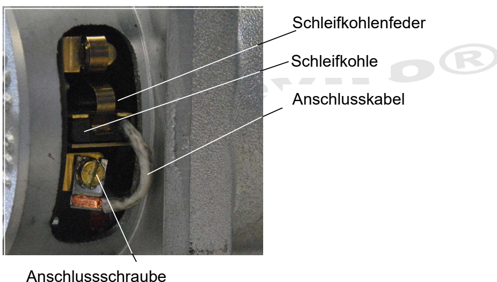
Abbildung 7 Schleifkohlenaustausch
