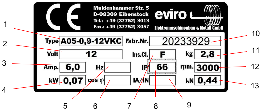
Abbildung 1 Typenschild
