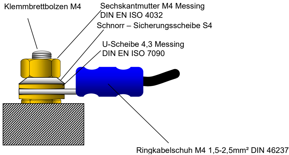
Abbildung 4 Ausführung der elektrischen Anschlüsse im Klemmkasten
