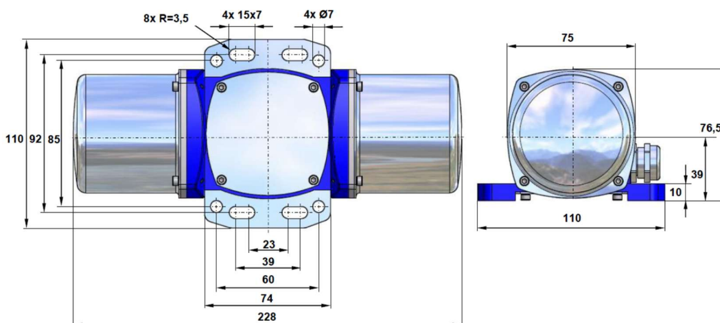
Abbildung 2 Abmaße
