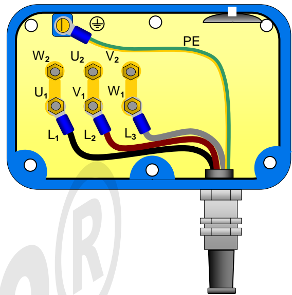
Abbildung 4 G31 Klemmkastenbelegung 3 ~ 230 V / Δ- Schaltung
