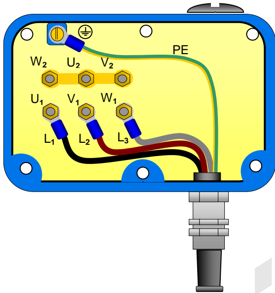
Abbildung 3 G31 Klemmkastenbelegung 3 ~ 400 V / Y- Schaltung
