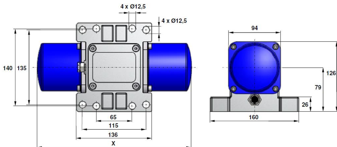
Abbildung 2 Abmaße
