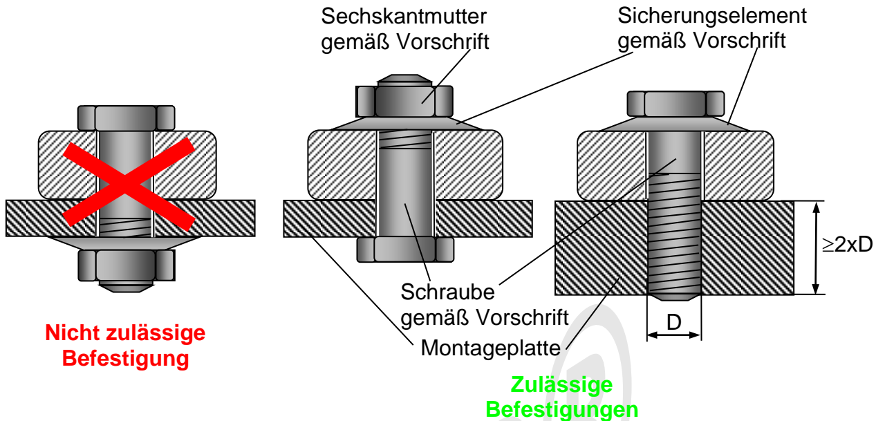
Abbildung 3 Befestigungsarten des Rüttelmotors
