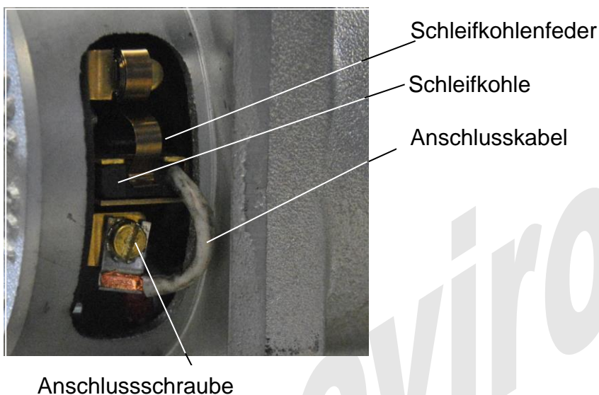
Abbildung 7 Schleifkohlenaustausch
