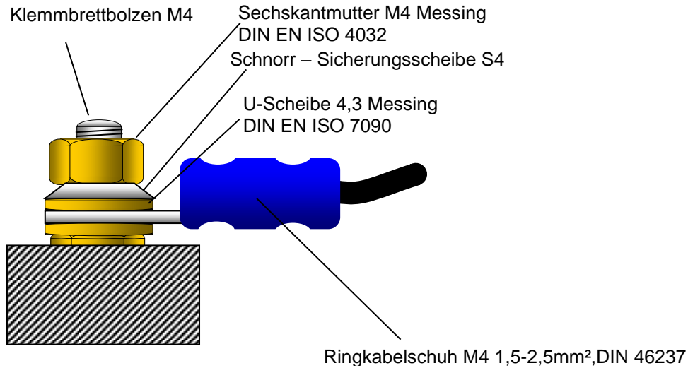
Abbildung 4 Ausführung der elektrischen Anschlüsse im Klemmkasten
