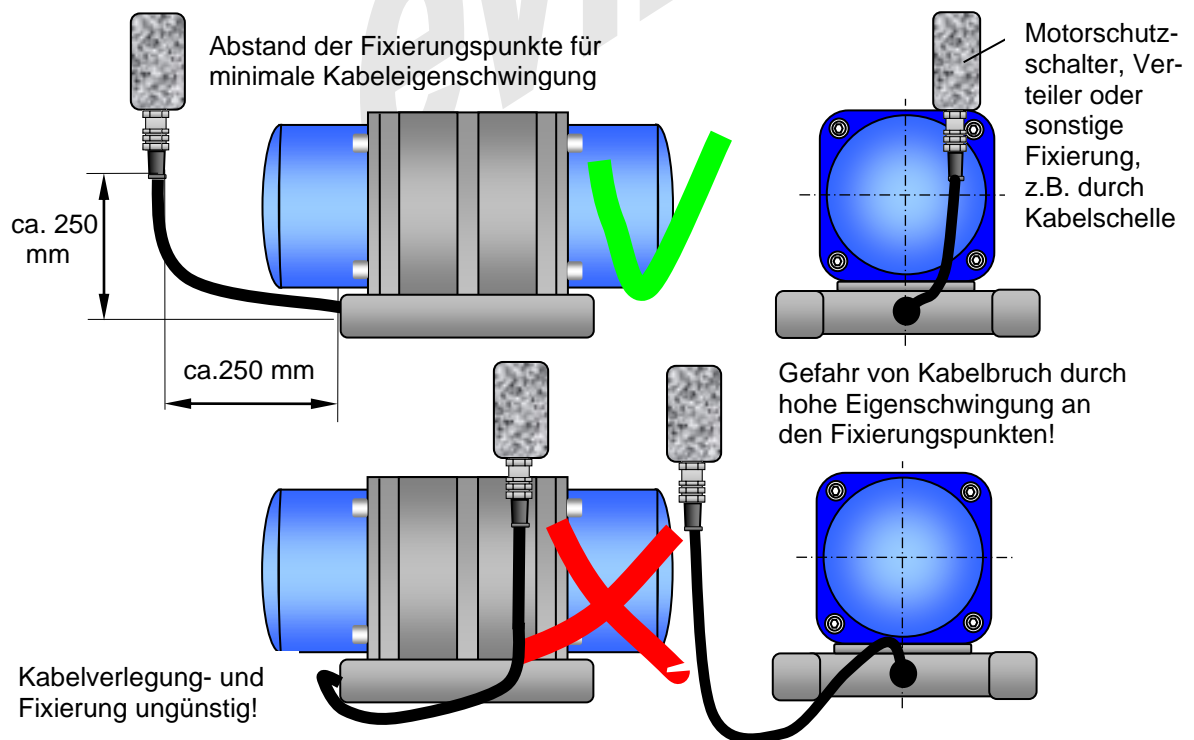
Abbildung 5 Kabelverlegung Anschlussleitung
