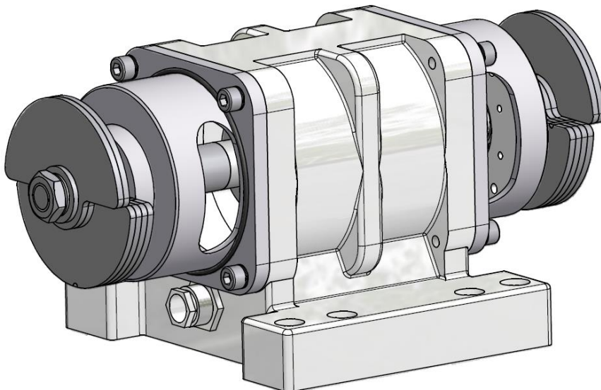
Abbildung 6 Einstellung der Fliehscheiben
